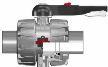
Шаровой кран промышленного применения VKD ХПВХ с втулочными окончаниями, DN65-100 d90 (DN80)
