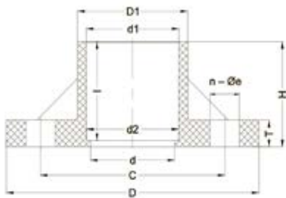
Жесткий фланец ХПВХ IPS (Model A) d63 PN16
