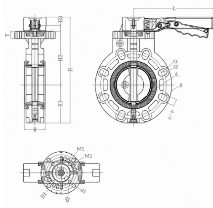
Затвор дисковый в корпусе FRPP (диск - ХПВХ) с рукояткой промышленного применения EPDM IPS d63 (DN50)
