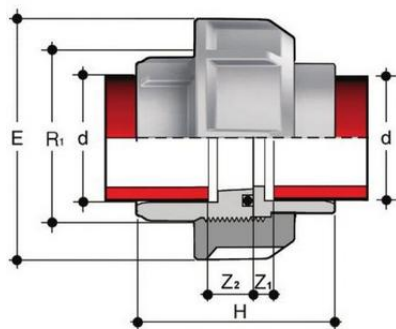
Муфта разборная для раструбной сварки PP-H FIP d20 PN10
