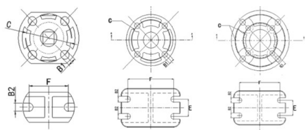
Шаровой кран IVKD PBX с эл.приводом 220V AC, муфтовые окончания, EPDM, IPS d63 (DN50)
