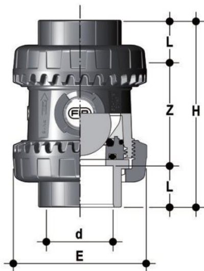
Шаровой обратный клапан SXEIV ПВХ; с муфтовыми окончаниям, EPDM, FIP d20 (DN15)
