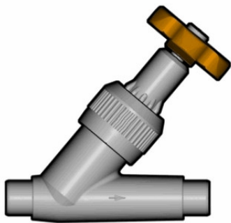
Угловой вентиль VVDV ПВХ с втулочными окончаниями, EPDM, FIP d50 (DN40)
