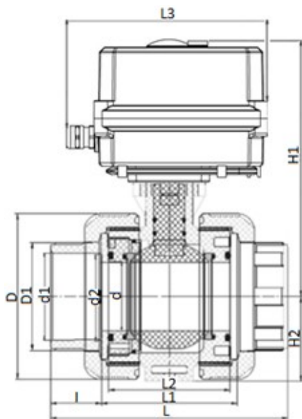
Шаровой кран IVKD ПВХ с эл.приводом 24V DC, муфтовые окончания, FKM, IPS d50 (DN40)
