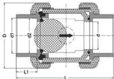
Шаровой обратный клапан ISXE ПВХ; с муфтовыми окончаниям, FKM, IPS d63 (DN50)
