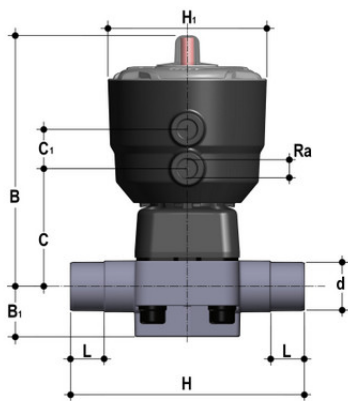
Мембранный клапан DK с пневмоприводом НЗ, PN10 с втулочными окончаниями (уплотнение EPDM/мембрана EPDM) PP-H d63 (DN50)
