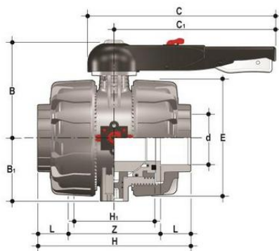
Шаровой кран промышленного применения VKD ХПВХ с муфтовыми окончаниями, DN65-100 d90 (DN80)
