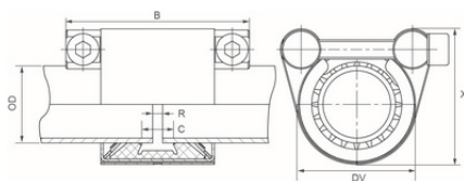
Соединительная муфта GRIP Ø25.0-48.3, FKM, W5 d28
