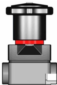
Компактный мембранный клапан CM ПВХ с пневмоприводом НЗ, муфтовые окончания, EPDM, FIP d16 (DN10)
