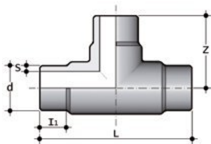
Тройник равнопроходной для стыковой сварки PP-H FIP (PN10) d355 SDR11 PN10
