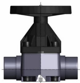
Мембранный клапан VM ПВХ с втулочными окончаниями d110 (DN90)
