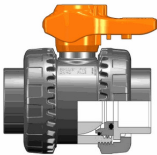
Шаровой кран общего применения VXE ХПВХ с муфтовыми окончаниями d20 (DN15)
