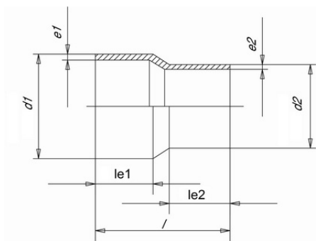
Муфта редукционная ПВДФ (Simona) 140x125 SDR33 PN10
