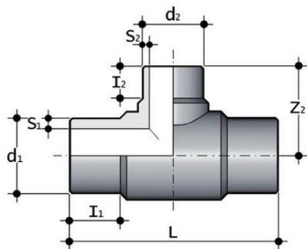
Тройник редукционный для стыковой сварки PP-H FIP (PN10) 90x75 SDR11 PN10
