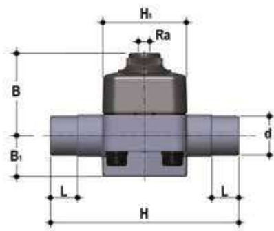
Мембранный клапан PBX с пневмоприводом прямого действия, DK, EPDM, FIP d25 (DN20)
