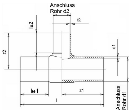
Тройник редукционный PP-H Simona (PN10) 63x50 SDR11 PN10
