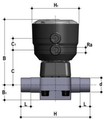
Мембранный клапан DK с пневмоприводом НЗ, PN6 с втулочными окончаниями (уплотнение EPDM/мембрана EPDM) PP-H d40 (DN32)
