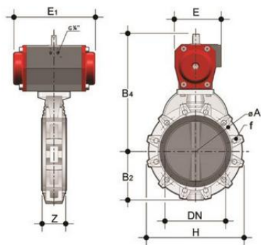
Дисковый затвор промышленного применения FK ПВХ с пневмоприводом НЗ, FKM, FIP d280 (DN250)
