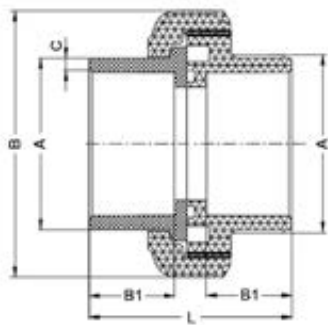
Муфта разборная для стыковой сварки PP-H IPS d75 PN 10
