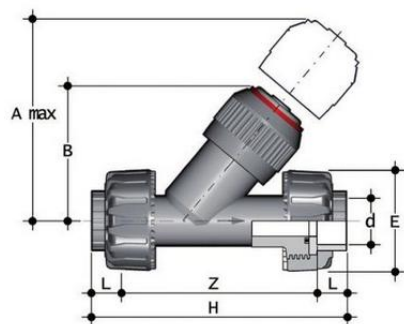
Угловой обратный клапан VRUIV ПВХ с разборными муфтовыми окончаниями, EPDM, FIP d25 (DN20)
