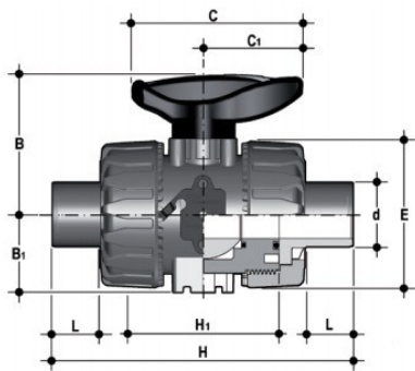
Шаровой кран промышленного применения VKD ХПВХ со втулочными окончаниями d20 (DN15)
