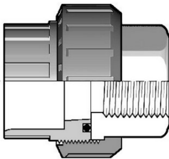
Муфта разборная переходная ХПВХ/ нержавеющая сталь ВР 16х3/8" PN16
