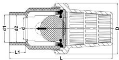
Донный клапан IVZ ПВХ с муфтовыми окончаниями, EPDM, FIP d40 (DN32)
