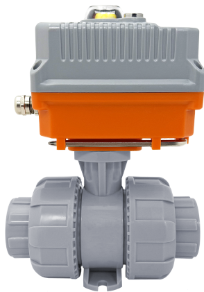
Шаровой кран IVKD ХПВХ с эл.приводом 24V DC, муфтовые окончания d63 (DN50)
