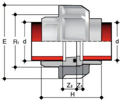
Муфта разборная ПВХД d20 SDR21 PN16
