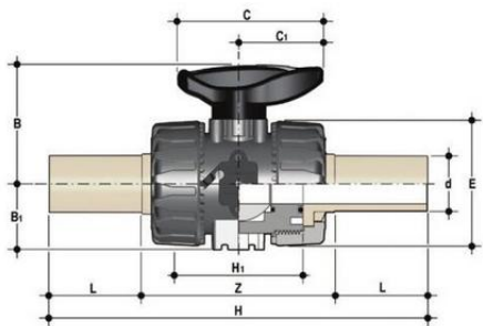
Шаровой кран промышленного применения VKD с патрубками (CVDM) (уплотнение EPDM) PP-H d25 (DN20)
