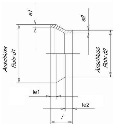
Муфта редукционная PP-H Simona 110x63 SDR11 PN6
