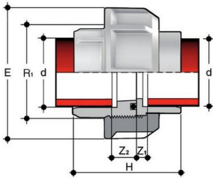
Муфта разборная ПВДФ d40 SDR21 PN16
