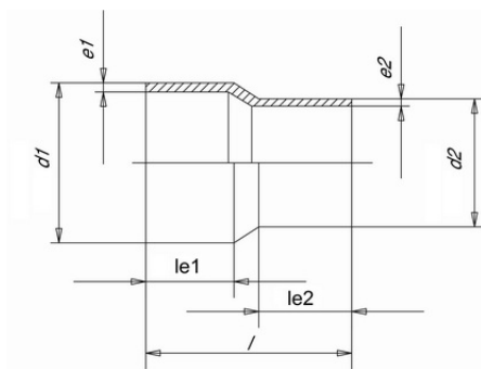
Муфта редукционная ПВДФ (Simona) 110x90 SDR33 PN10
