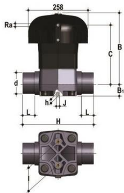
Мембранный клапан ПВХ с пневмоприводом, VM, FKM, FIP d110 (DN100)
