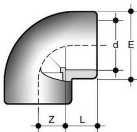
Отвод клеевой 90° ПВХ FIP d16
