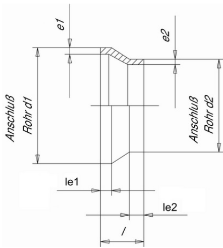
Муфта редукционная ПВДФ (Simona) 125x110 SDR21 PN16
