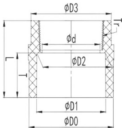
Муфта переходная с ВР ПВХ IPS 110x4"
