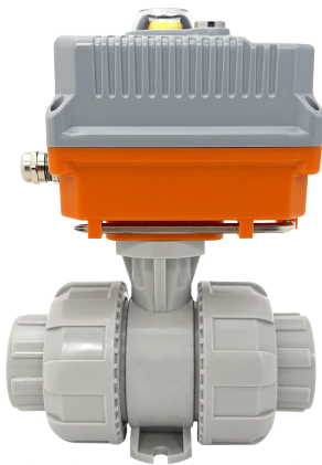
Шаровой кран IVKD ПП-гомополимер с эл.приводом 220V AC, муфтовые окончания, EPDM, IPS d90 (DN80)
