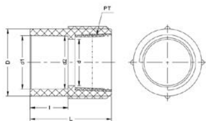
Муфта ХПВХ IPS 63x2" PN16
