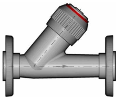
Угловой обратный клапан VROV ПВХ с фланцевыми окончаниями, FKM, FIP d25 (DN20)
