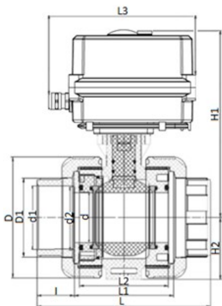
Шаровой кран IVKD ПВХ с эл.приводом 24V DC, муфтовые окончания, FKM, IPS d20 (DN15)
