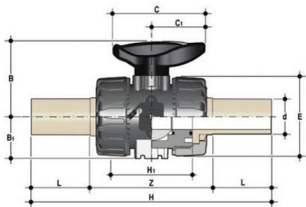
Шаровой кран промышленного применения VKD с патрубками (CVDM) (уплотнение EPDM) PP-H d25
