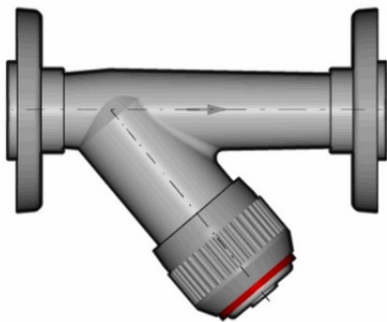
Грязевый фильтр RVOT ПВХ с фланцевыми окончаниями, EPDM, FIP d32 (DN25)
