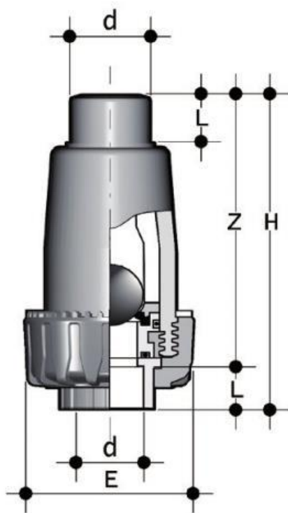
Шаровой обратный клапан SR с муфтовыми окончаниями (уплотнение FKM) PP-H d50 (DN40)
