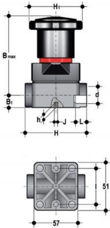
Компактный мембранный клапан ПВХ с пневмоприводом, CM, EPDM, FIP d16 (DN10)
