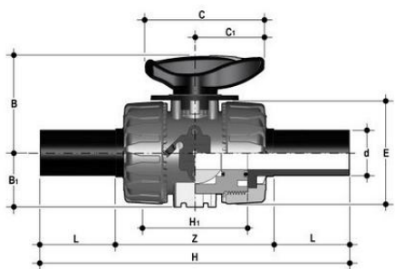
Шаровой кран для регулирования потока VKR с партрубками из ПЭ (уплотнение FKM) PP-H d50 (DN40)
