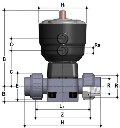
Мембранный клапан ДК ХПВХ с пневмоприводом ДвД, PN10, разборные резьбовые окончания 1 1/4"
