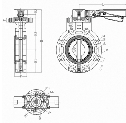
Затвор дисковый в корпусе FRPP (диск - НПВХ) с рукояткой промышленного применения FKM IPS 110 (DN100)
