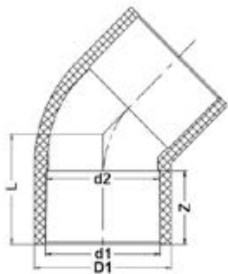
Отвод для раструбной сварки 45° PP-H IPS d110 PN10
