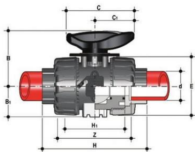
Шаровой кран для регулирования потока VKRIM с муфтовыми окончаниями (уплотнение EPDM) PP-H d32 (DN25)
